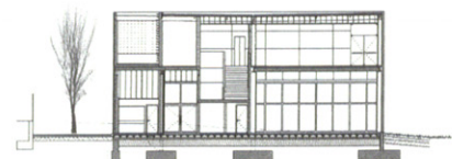
10 · SECCIONES TRANSVERSALES
